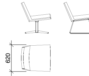
s251 modal
